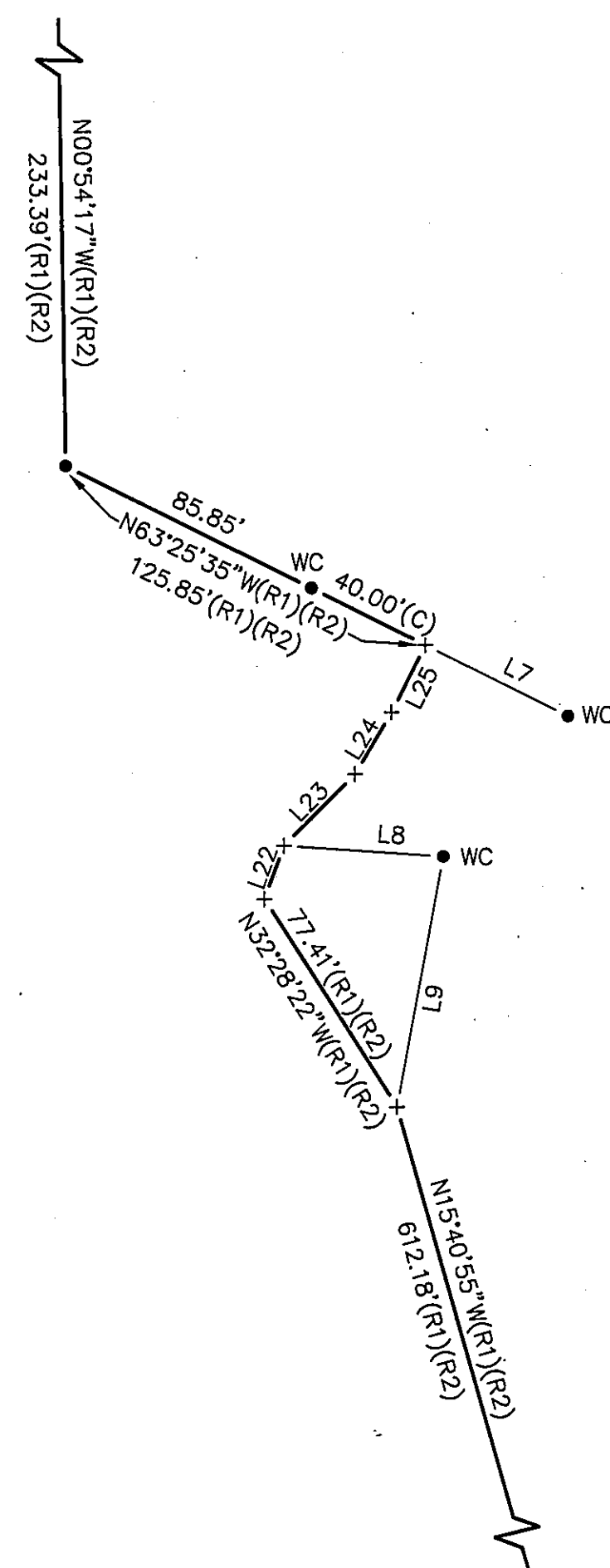
DETAIL 'B' SCALE: 1"=50'
